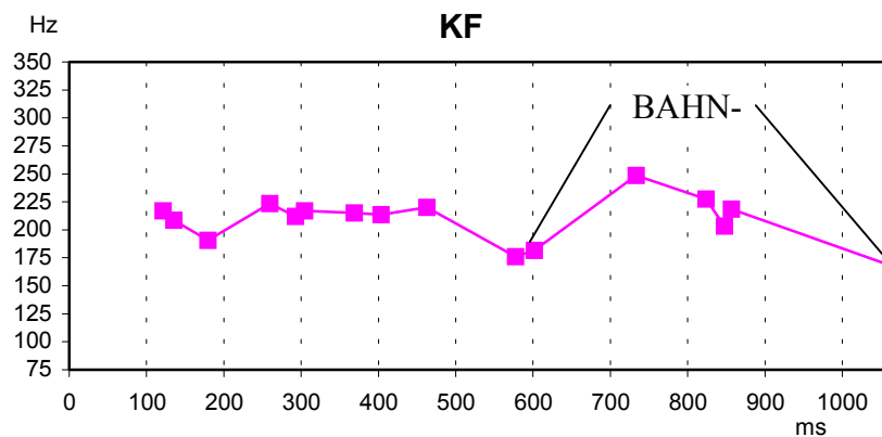
Abb. 4: Prototypische F0-Kontur (8 Sprecherinnen) des Satzes ‚Sie fuhr zum Bahnhof.‘, eingebettet in einen Kontrast auslösenden Kontext.
