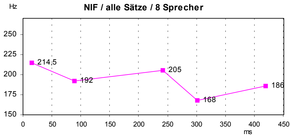
Abb. 5: Prototypische F0-Kontur in Kontext mit Neuinformationsfokus (8 Sprecherinnen, 8 Kontexte).
