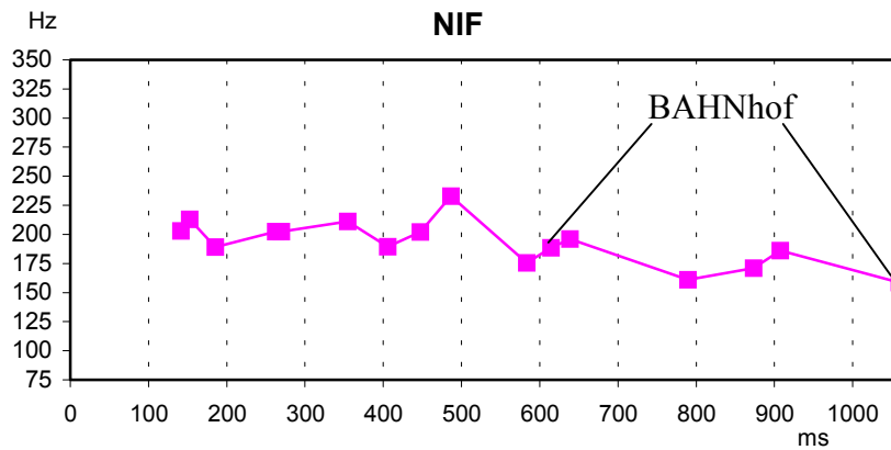
Abb. 3: Prototypische F0-Kontur (8 Sprecherinnen) des Satzes ‚Sie fuhr zum Bahnhof.‘ in Kontext mit Neuinformationsfokus.
