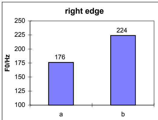
Abb. 8: absolute F0-Werte in der Umgebung der rechtsseitigen Begrenzung für NIF (a) und KF (b) der Zielkonstituente für alle Sprecher und alle Kontexte
