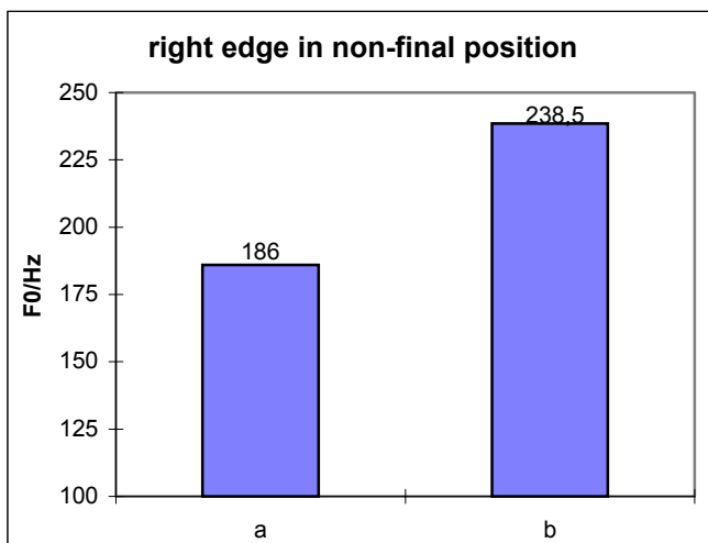
Abb. 9: absolute F0-Werte in der Umgebung der rechtsseitigen Begrenzung für NIF (a) und KF (b) der Zielkonstituenten, die in nicht-satzfinaler Position stehen
