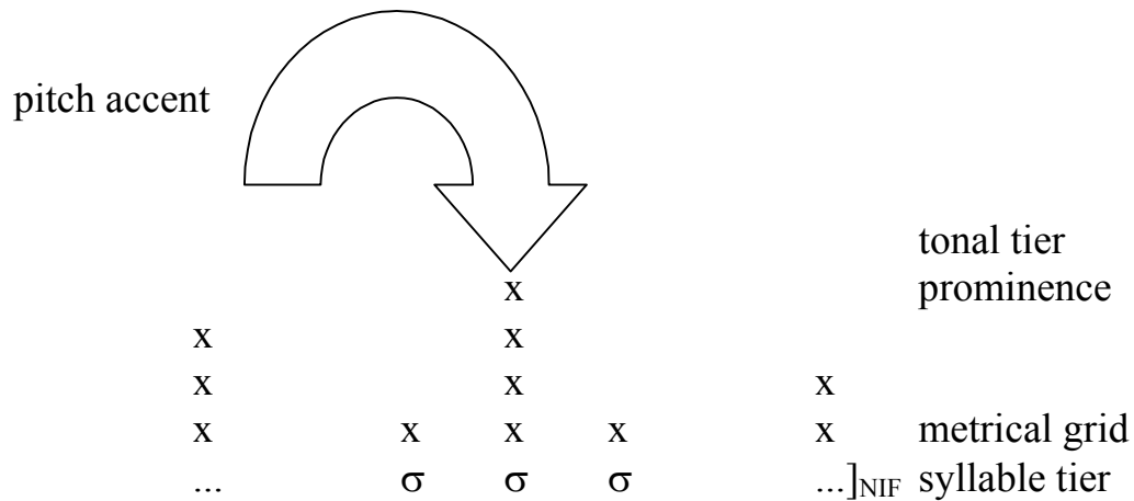
Abb. 10: (Default-) Satzakkent-Zuweisung
