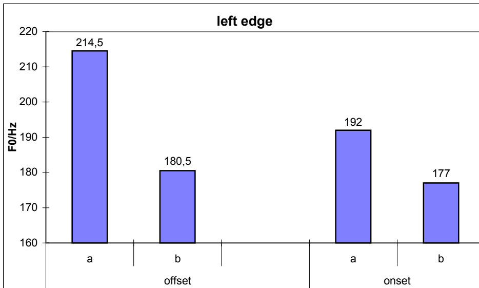
Abb. 7: absolute F 0 -Werte in der Umgebung der linksseitigen Begrenzung für NIF (a) und KF (b) der Zielkonstituente für alle Sprecher und alle Kontexte. Offset = rechte Begrenzung der Vorgängerkonstituente; Onset = Beginn der Zielkonstituente
