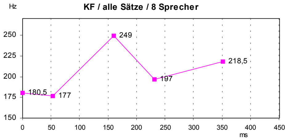
Abb. 6: Prototypische F0-Kontur in Kontext mit Kontrastfokus (8 Sprecherinnen, 8 Kontexte).
