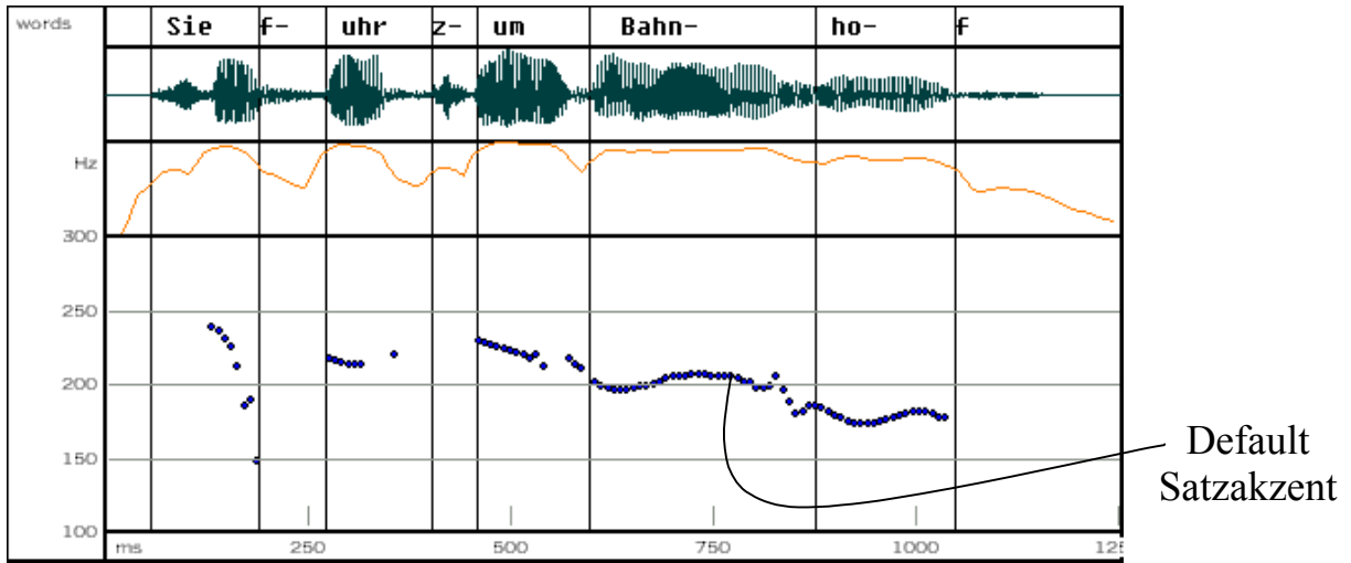
Abb. 1: Ein akustischer Einzelfall des Satzes ‚ Sie fuhr zum Bahnhof. ‘ im Kontext mit Neuinformationsfokus (1)(a).
