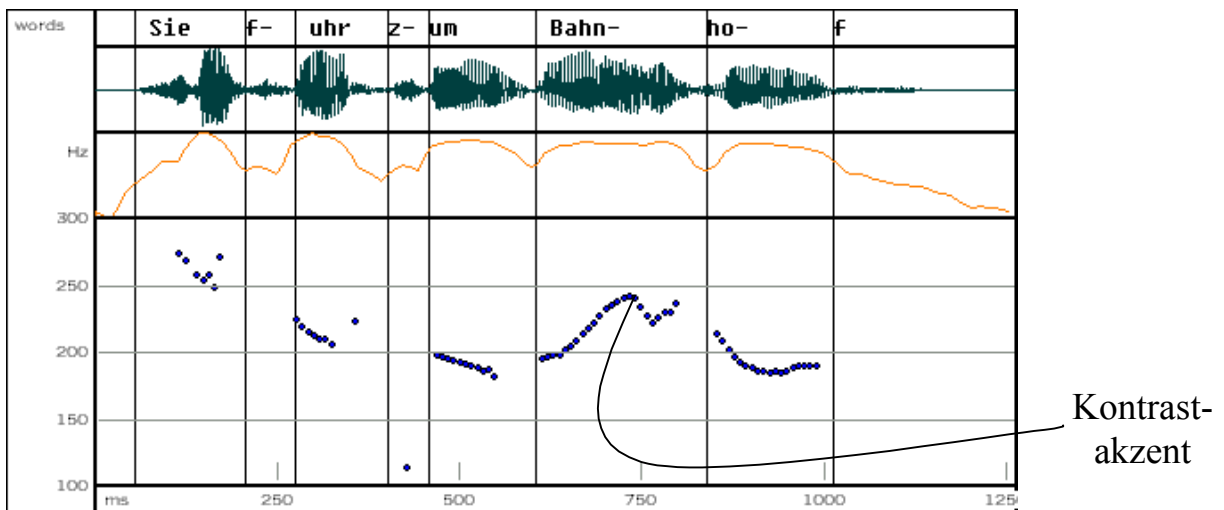
Abb. 2: Ein akustischer Einzelfall des Satzes ‚ Sie fuhr zum Bahnhof. ‘, eingebettet in einen Kontrast auslösenden Kontext (1)(b).
